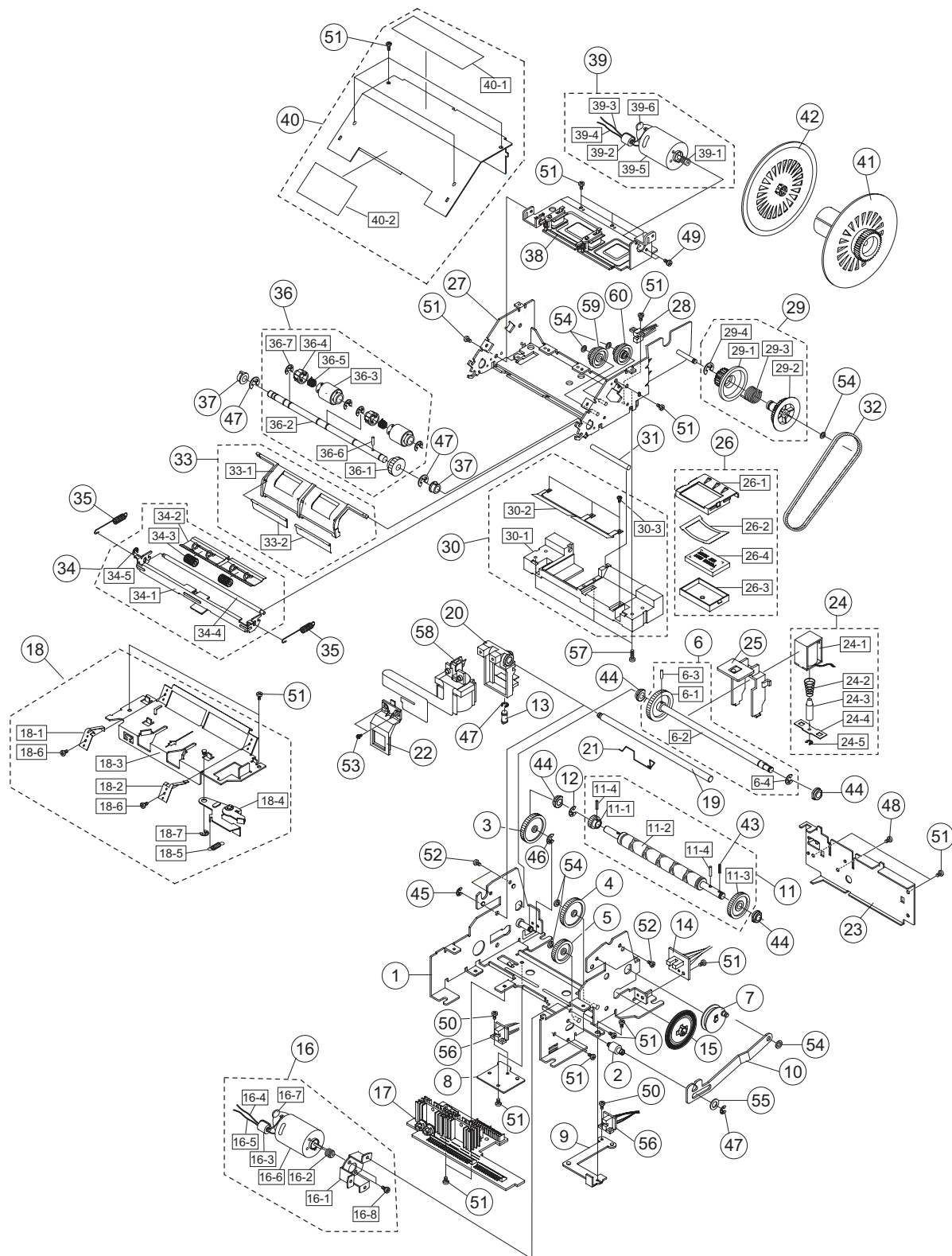
Figure7-5 Printer (ERP-400)
